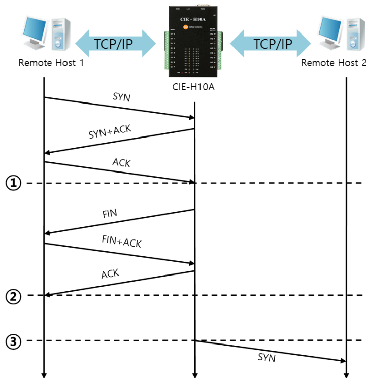
Схема 6-4 Временной график активации опции [TCP Server]
