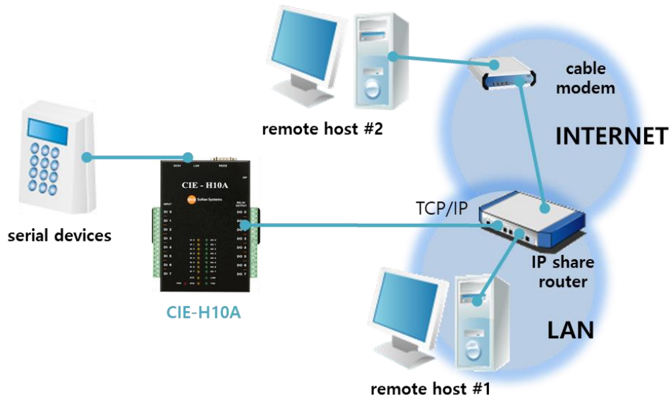
Схема 1-6 Сервер последовательных устройств
