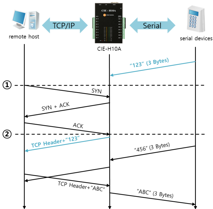
Схема 6-2 Временной график
