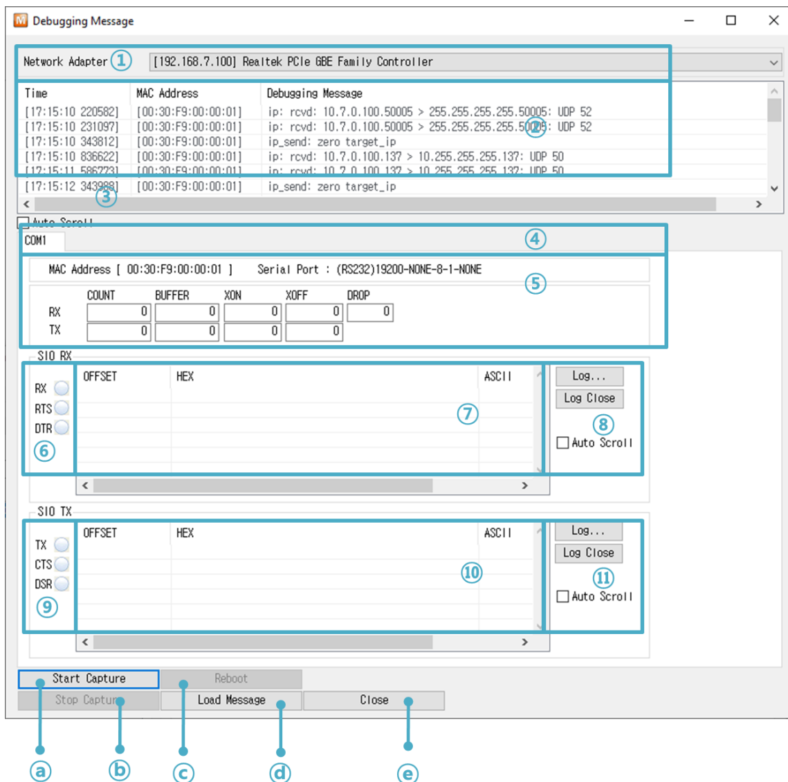
Схема 8-4 Окно сообщения отладки
