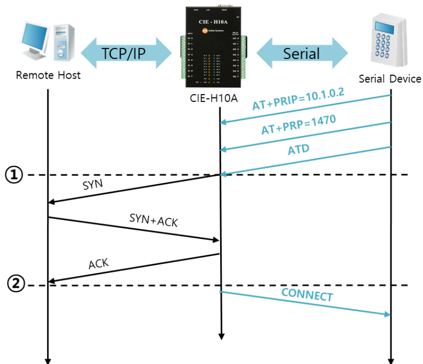
Схема 6-6 Активное TCP-соединение
