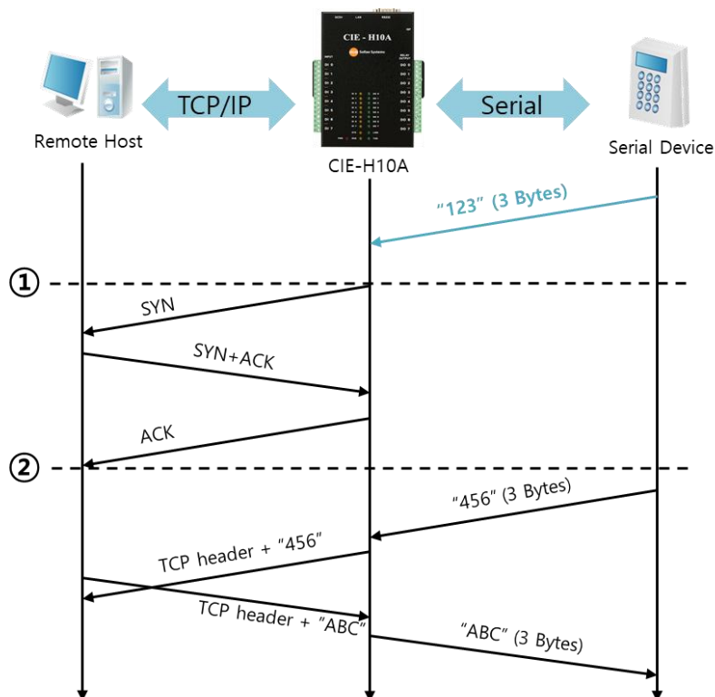
Схема 6-4 Временной график
