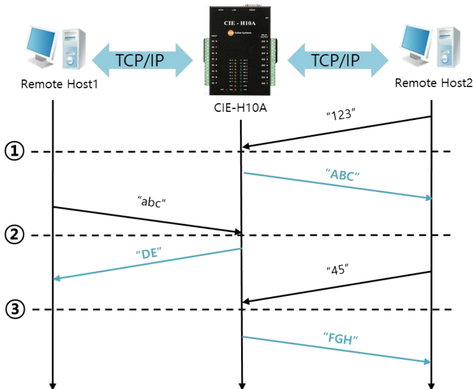
Схема 6-8 Временной график для [dynamic update of peer host]
