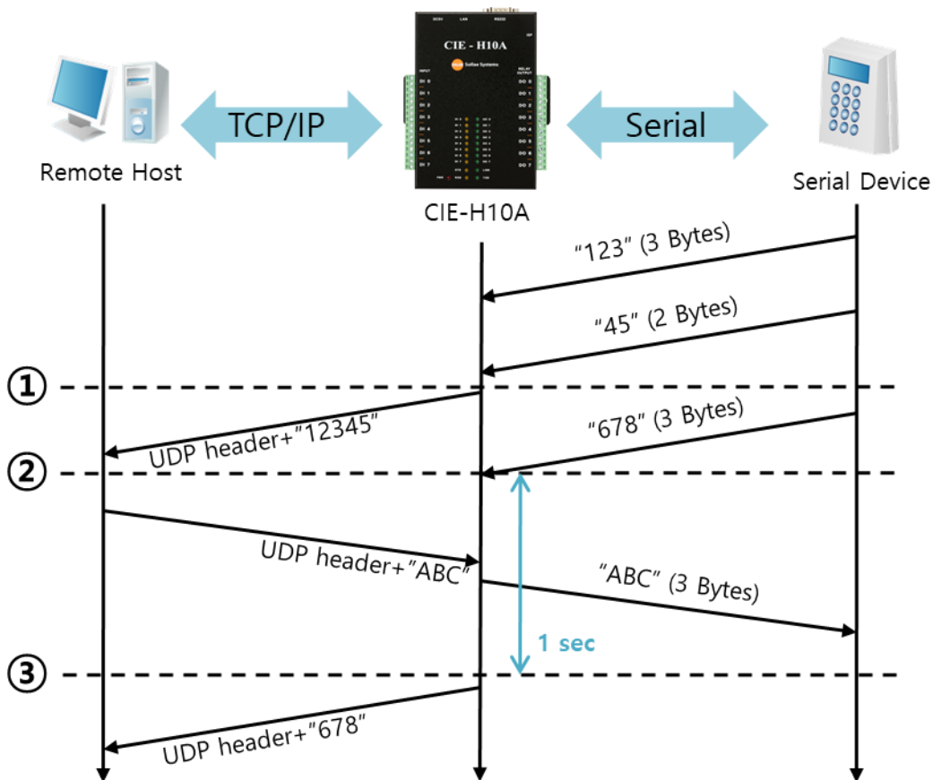
Схема 6-7 Временная диаграмма для размера блока составляет 5 байт, а интервал кадра данных равен 1 сек
