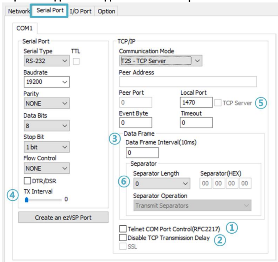
Схема 8-5 Вкладка последовательного порта
