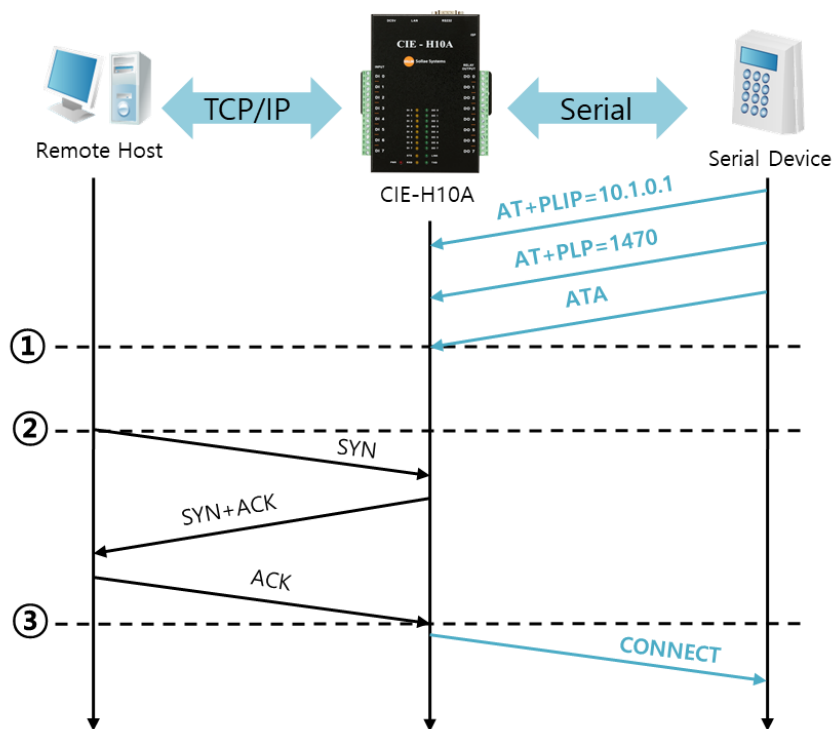
Схема 6-5 Пассивное TCP-соединение
