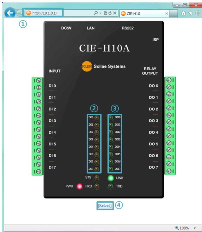
Схема 2-5 Тест HTTP
