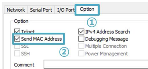
Схема 8-2 Настройка функции отправки MAC-адреса
