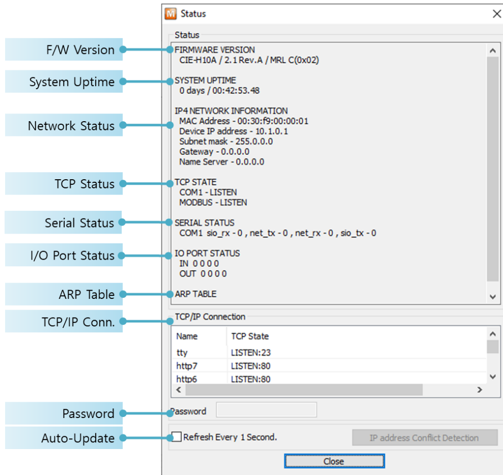
Схема 7-13 Окно состояния ezManager
