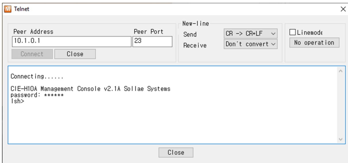
Схема 7-5 Вход в Telnet (ezManager)
