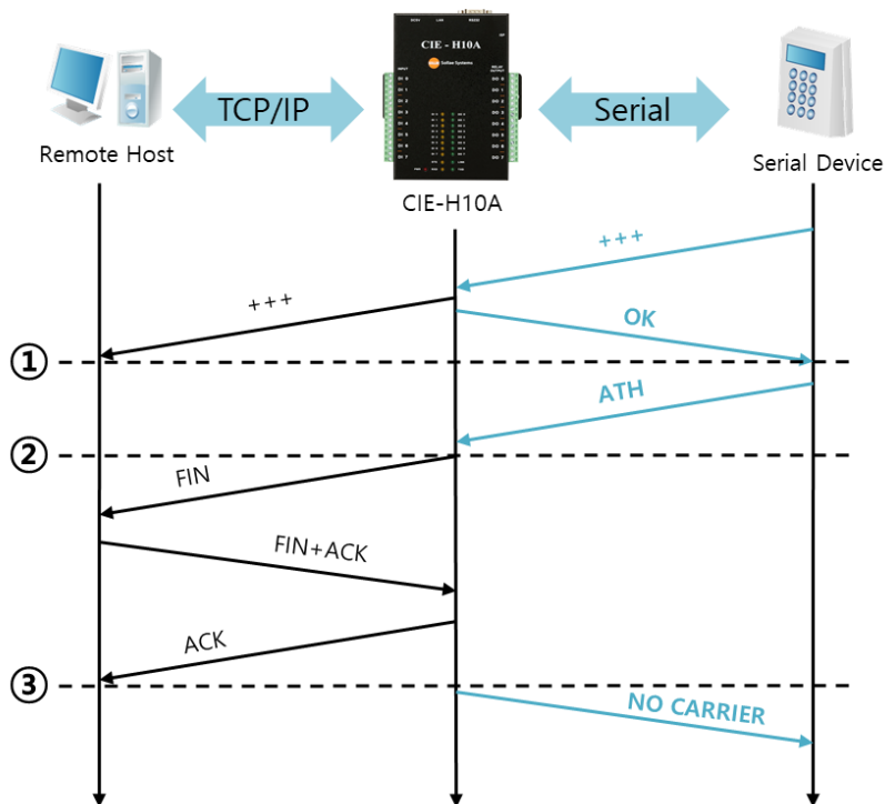
Схема 6-6 Временной график
