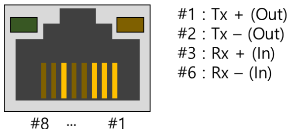
Схема 1-10 Разъем RJ45
