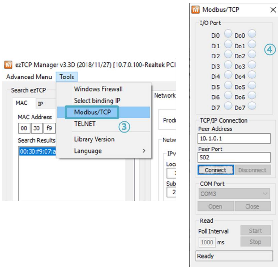
Схема 2-3 Тестовая Modbus/TCP программа в ezManager
