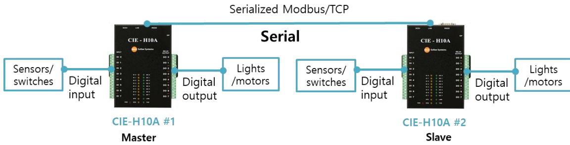
Схема 1-4 Последовательный коммутатор
