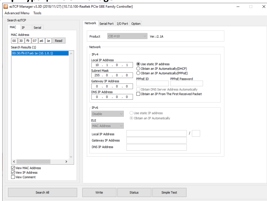
Схема 3-1 Главный экран ezManager
