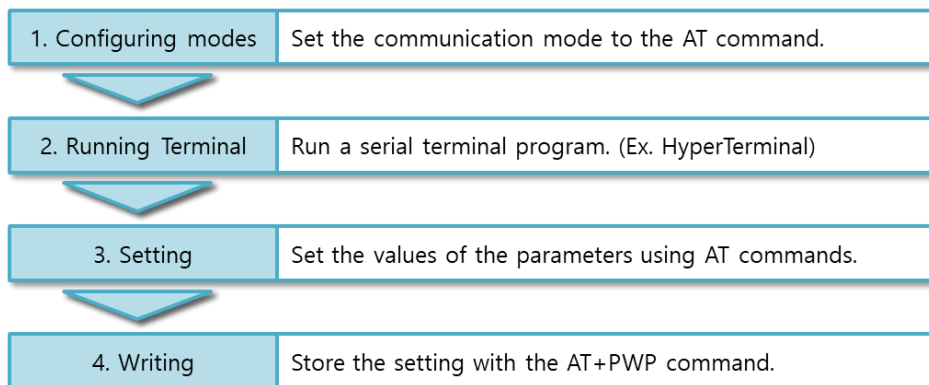
Схема 3-6 Процедуры конфигурации с АТ-командой
