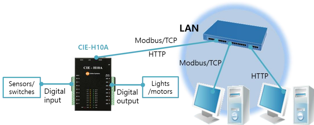
Схема 1-1 Сервер удаленного ввода/вывода
