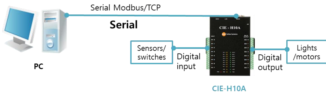
Схема 1-2 Последовательный Modbus/TCP
