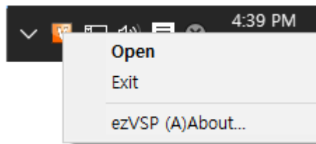
Fig. 3-2 Popup menus
