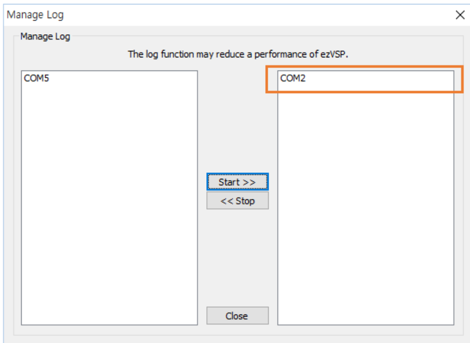
Fig. 3-20 Log (4)
