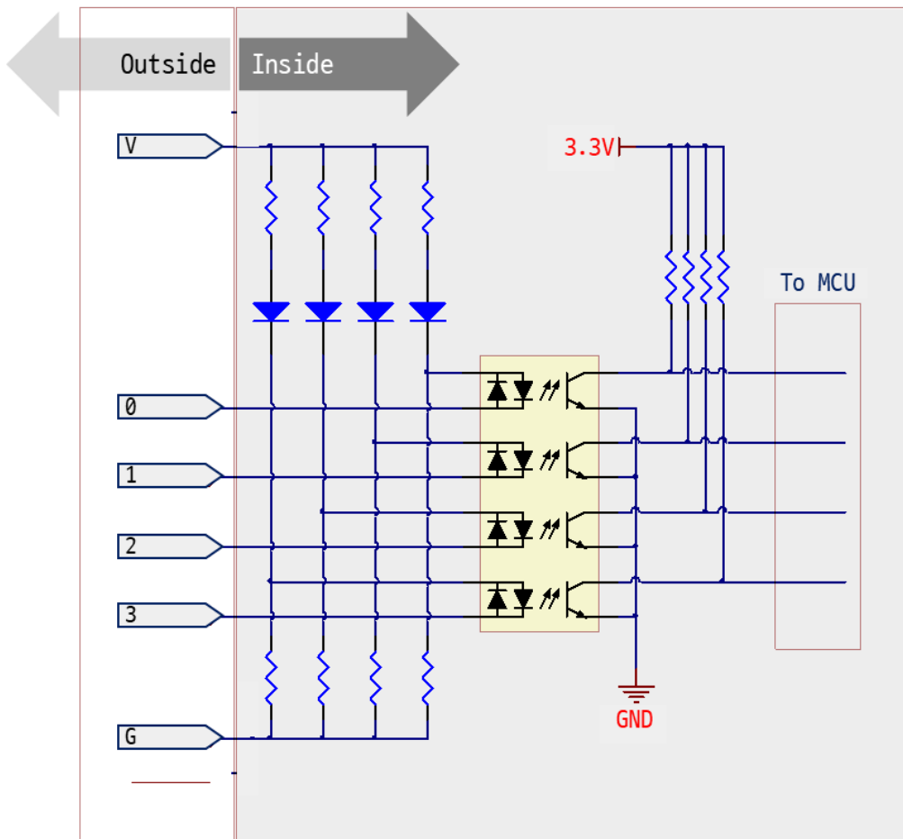
Схема 1-5 Схема цифрового входа
