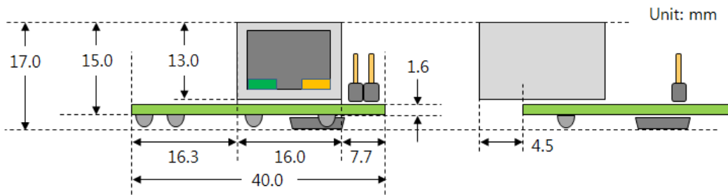
그림 1-7 정면도, 측면도
