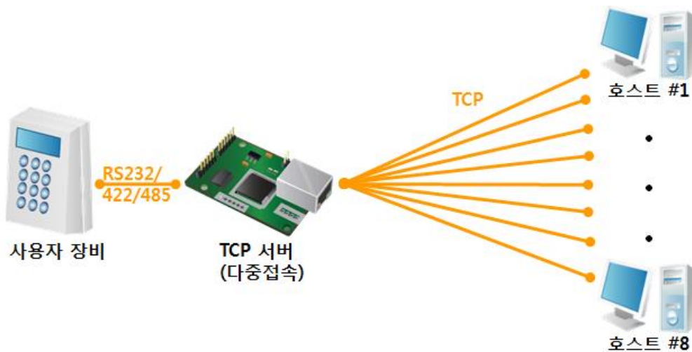
그림 7-10 다중 접속 개념도
