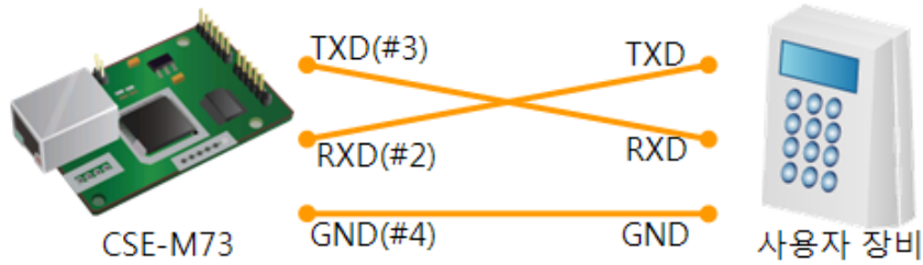
그림 8-1 올바른 RS232 연결 (JP1, 2)
