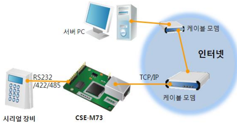
그림 1-3 케이블 모뎀에 적용한 구성
