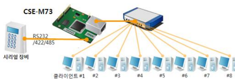
그림 1-5 다중 접속 적용 구성 예
