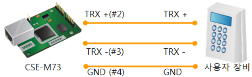
그림 8-3 올바른 RS485 연결 (JP4, 5)
