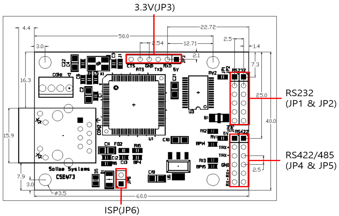
그림 1-6 CSE-M73 치수
