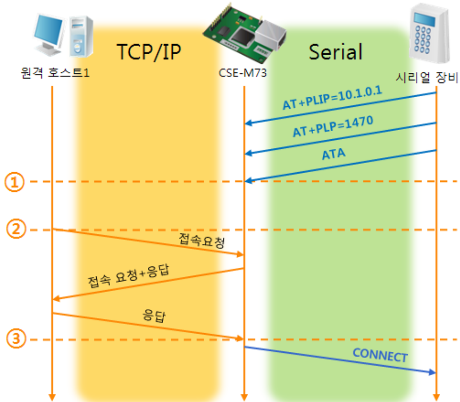
그림 5-7 TCP 수동접속
