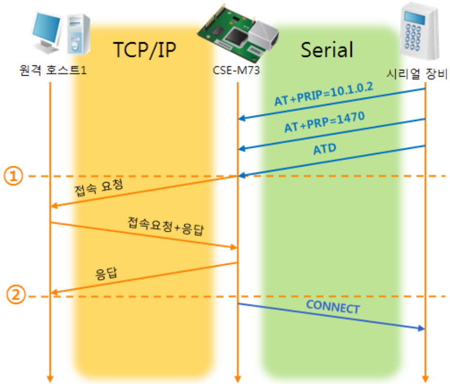
그림 5-8 TCP 능동접속
