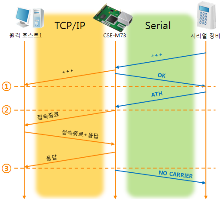
그림 5-9 TCP 접속종료
