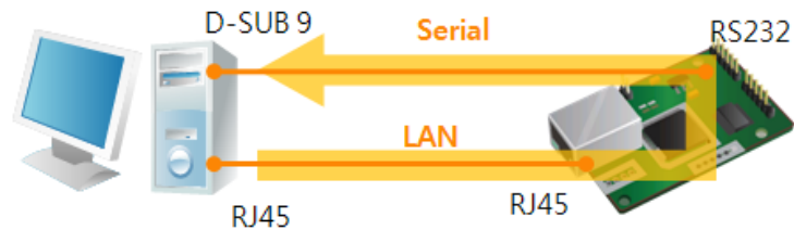
그림 2-8 LAN → RS232
