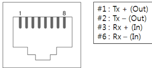
그림 1-8 RJ45 이더넷 커넥터 사양
