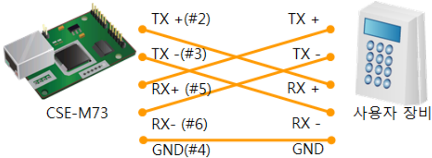
그림 8-2 올바른 RS422 연결 (JP4, 5)
