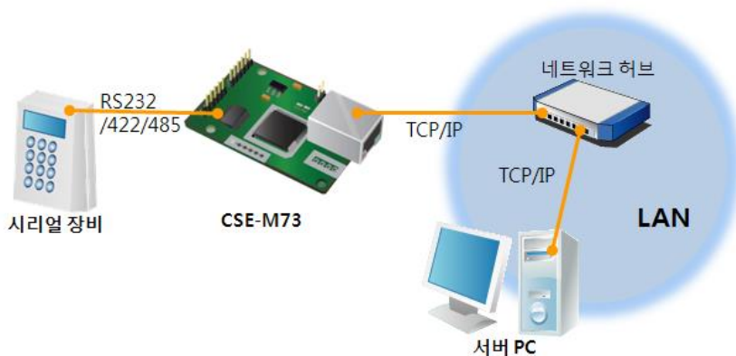
그림 1-2 LAN에 적용한 구성
