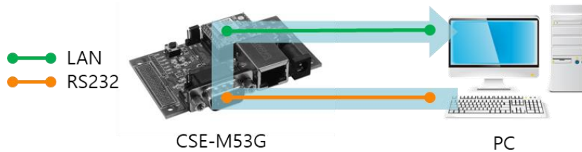
그림 2-9 RS232 → LAN
