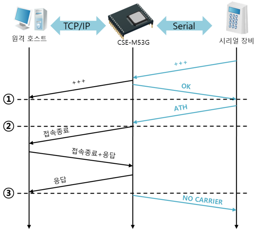
그림 5-9 TCP 접속종료
