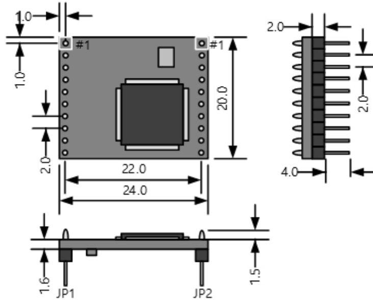
그림 1-6 CSE-M53G 치수
