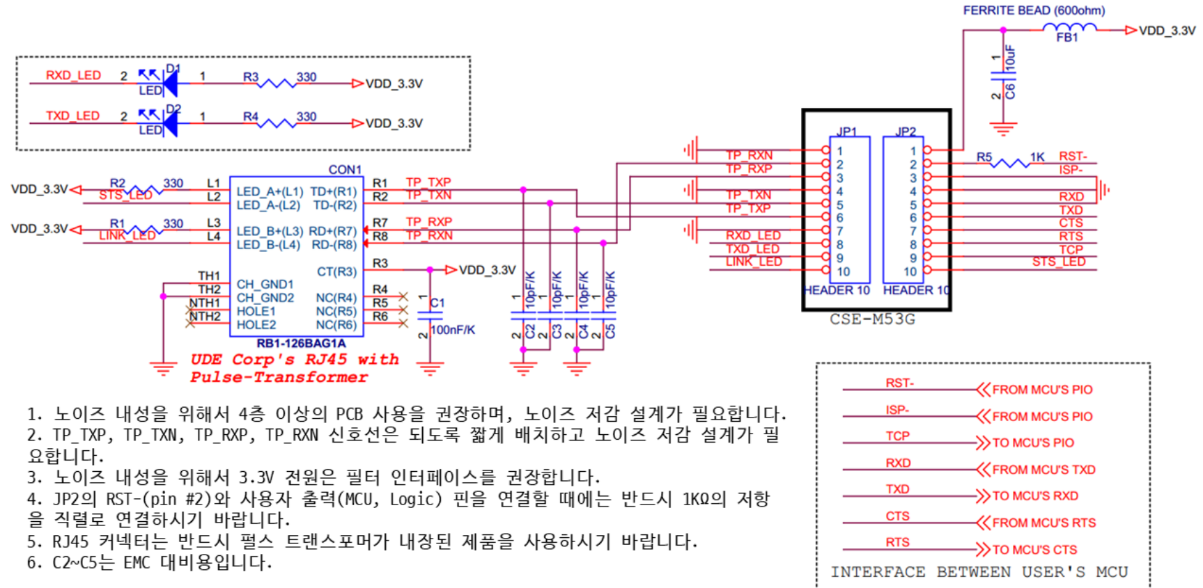
그림 1-7 응용 회로도
