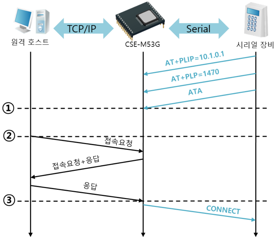
그림 5-7 TCP 수동접속
