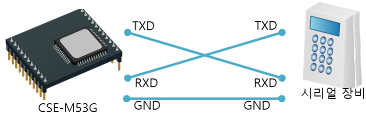
그림 9-1 올바른 RS232 연결
