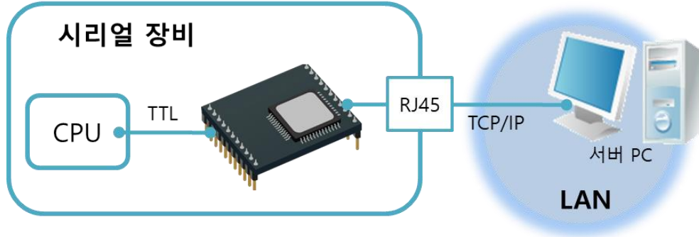
그림 1-1 PC와 1:1 연결
