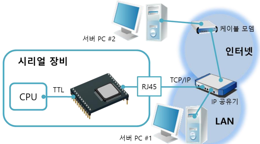
그림 1-4 IP공유기를 이용한 구성 예
