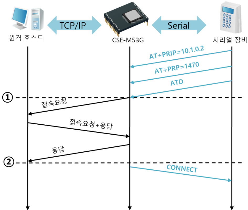
그림 5-8 TCP 능동접속
