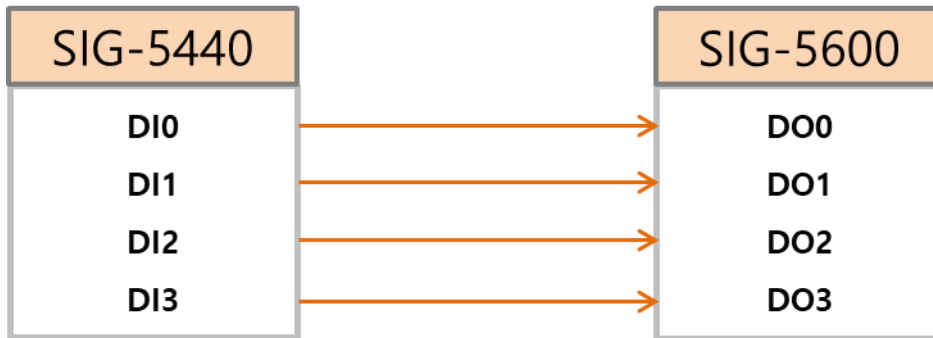
그림 2-2 마스터의 출력 제어
