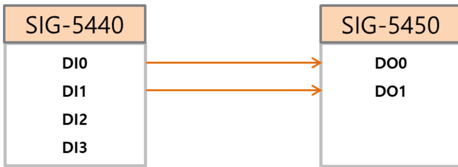
그림 2-6 마스터의 출력 제어
