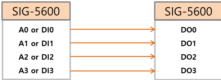
그림 2-3 마스터의 출력 제어
