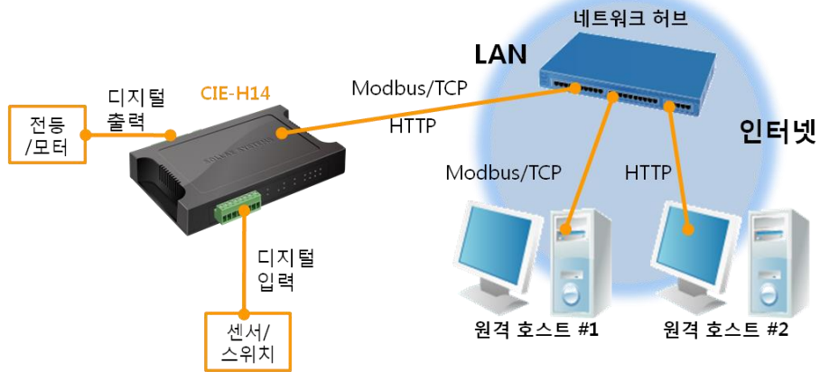
그림 1-1 원격 디지털 입/출력 감시/제어 구성 예
