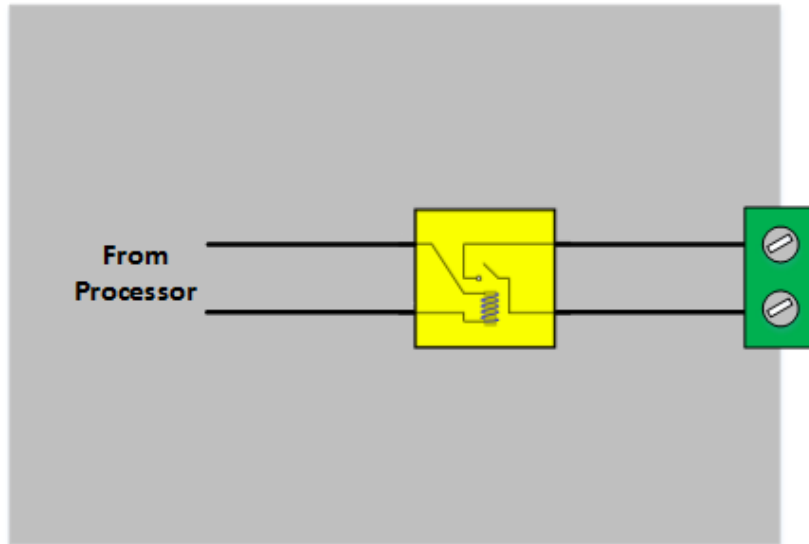
그림 1-9 출력포트 회로도
