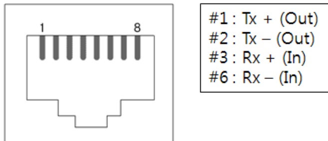
그림 1-12 RJ45 이더넷 커넥터 사양
