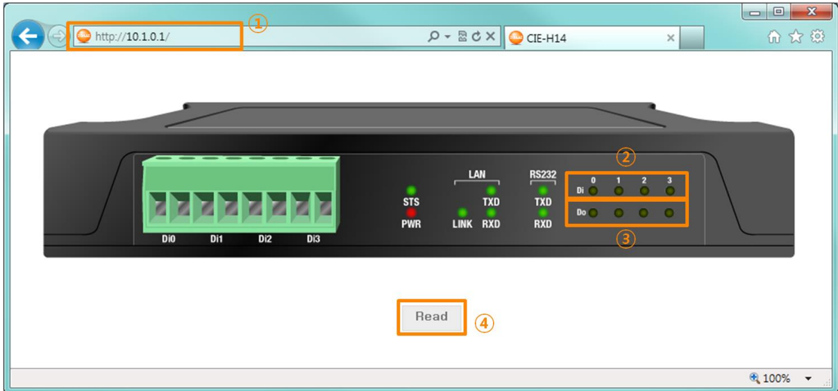
그림 2-5 웹 브라우저를 통한 접속 화면
