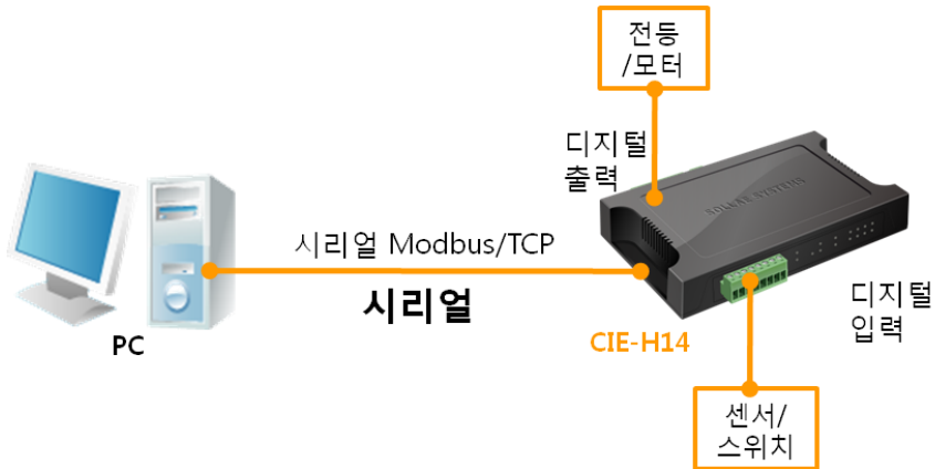
그림 1-2 시리얼 Modbus/TCP 구성 예
