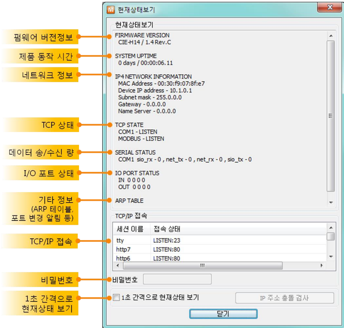
그림 7-14 ezManager의 현재상태보기 창
