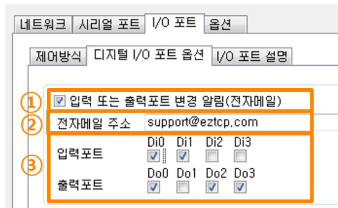
그림 8-6 입출력 포트 변경 알림 설정
