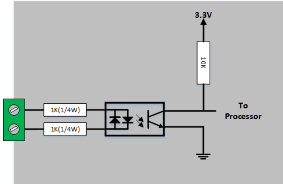
그림 1-8 입력 포트 회로도
