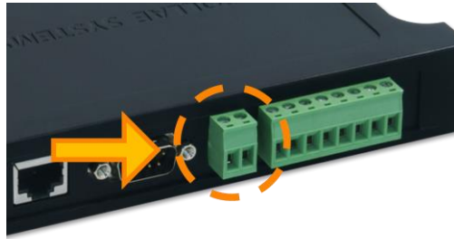
그림 1-7 전원
