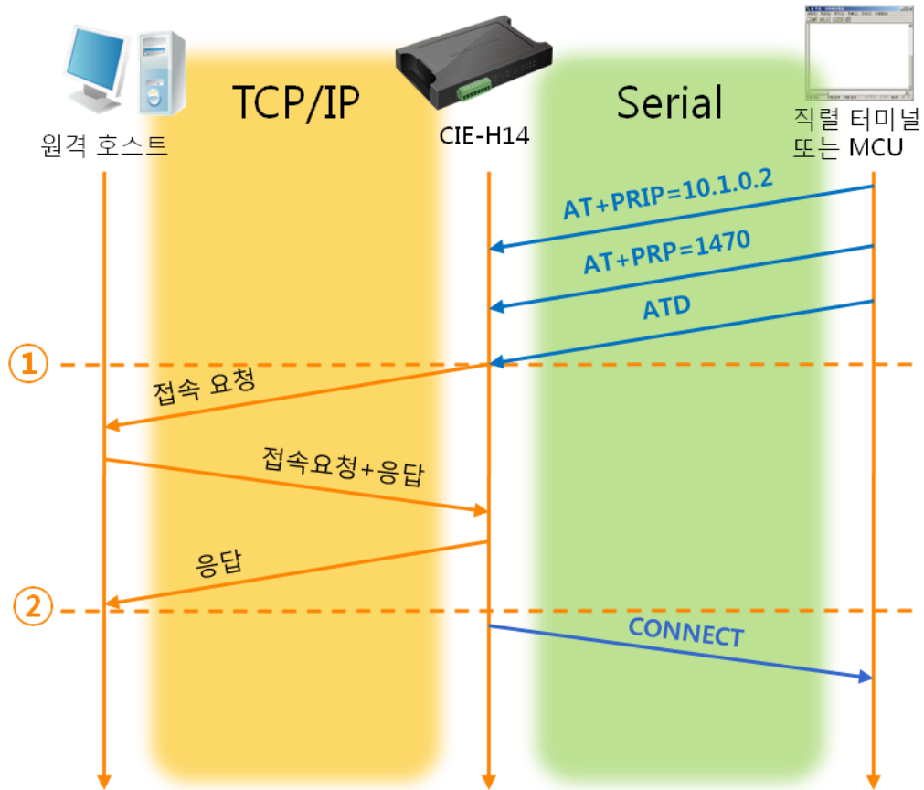
그림 6-5 TCP 능동접속
