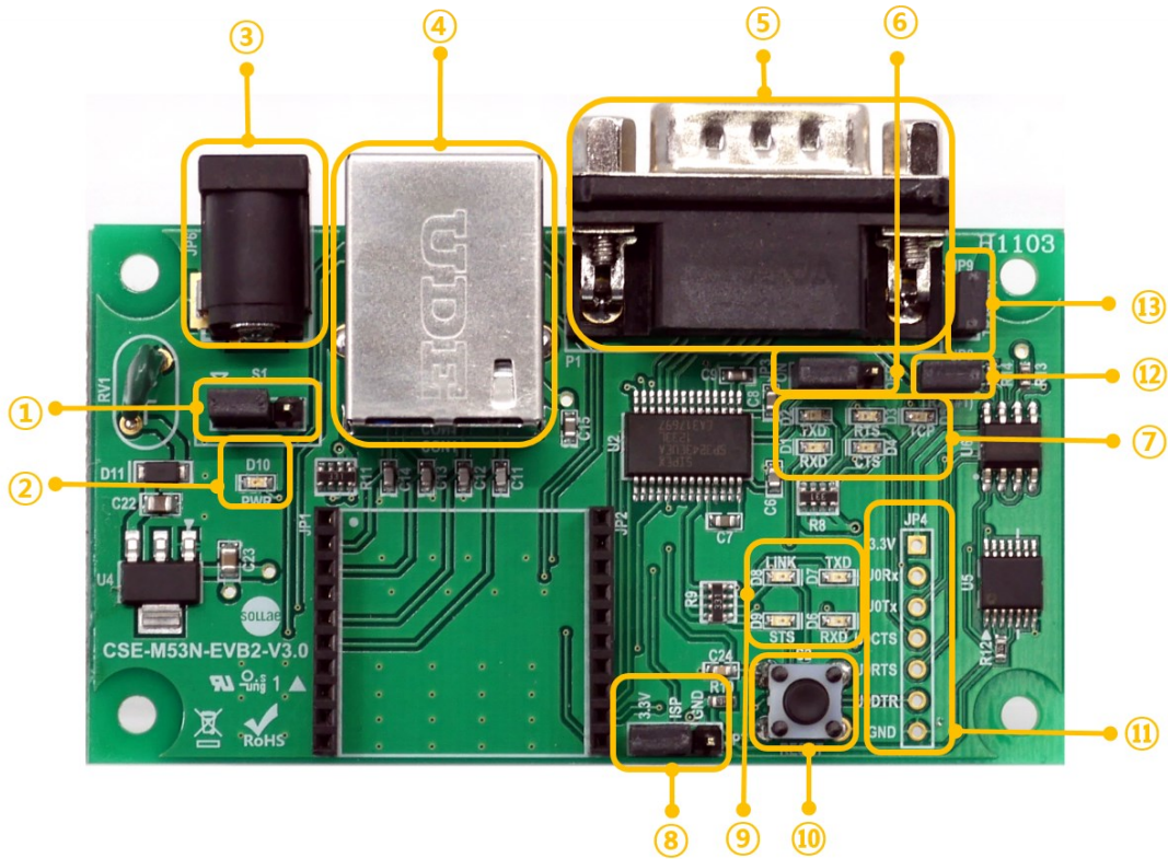
그림 1-2 CSE-M53/M53N-EVB2 실사
