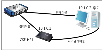
통신 테스트를 위한 연결 구성
