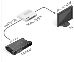
[CIE-H14A 설정 연결구성]
